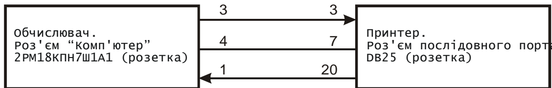
Рис. 5 Схема розпайки кабеля для з'єднання обчислювача і принтера
